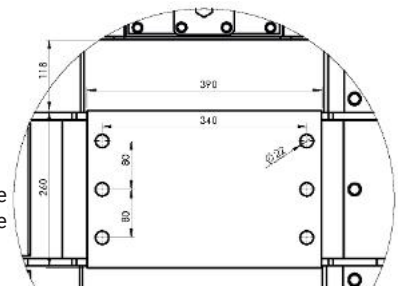
Anschlußmaße Kopfplatte für Terra-Star® Ecoline
